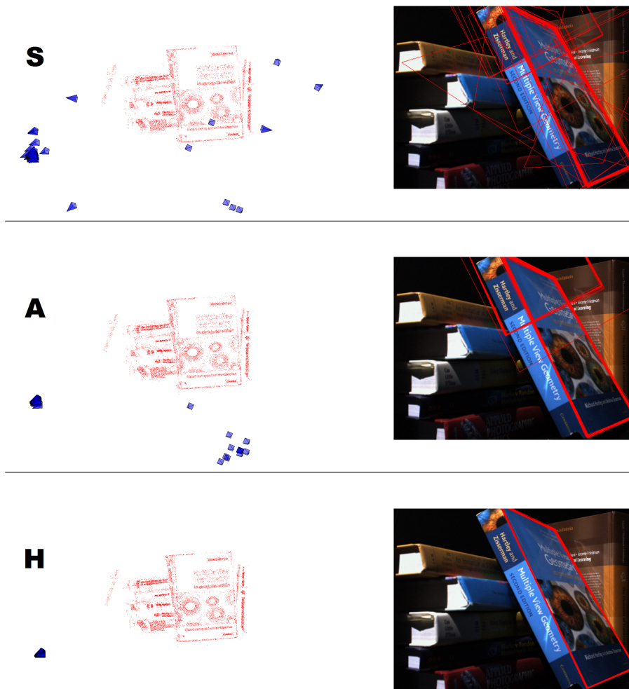
Figure 9. Séquence Livre : 100 poses calculées avec N = 1000 itérations de RANSAC, et la reprojection des bords de la couverture en utilisant ces 100 poses. Dans le scénario H l'écart-type de la position de la caméra est 0,29% de la distance à la scène.
