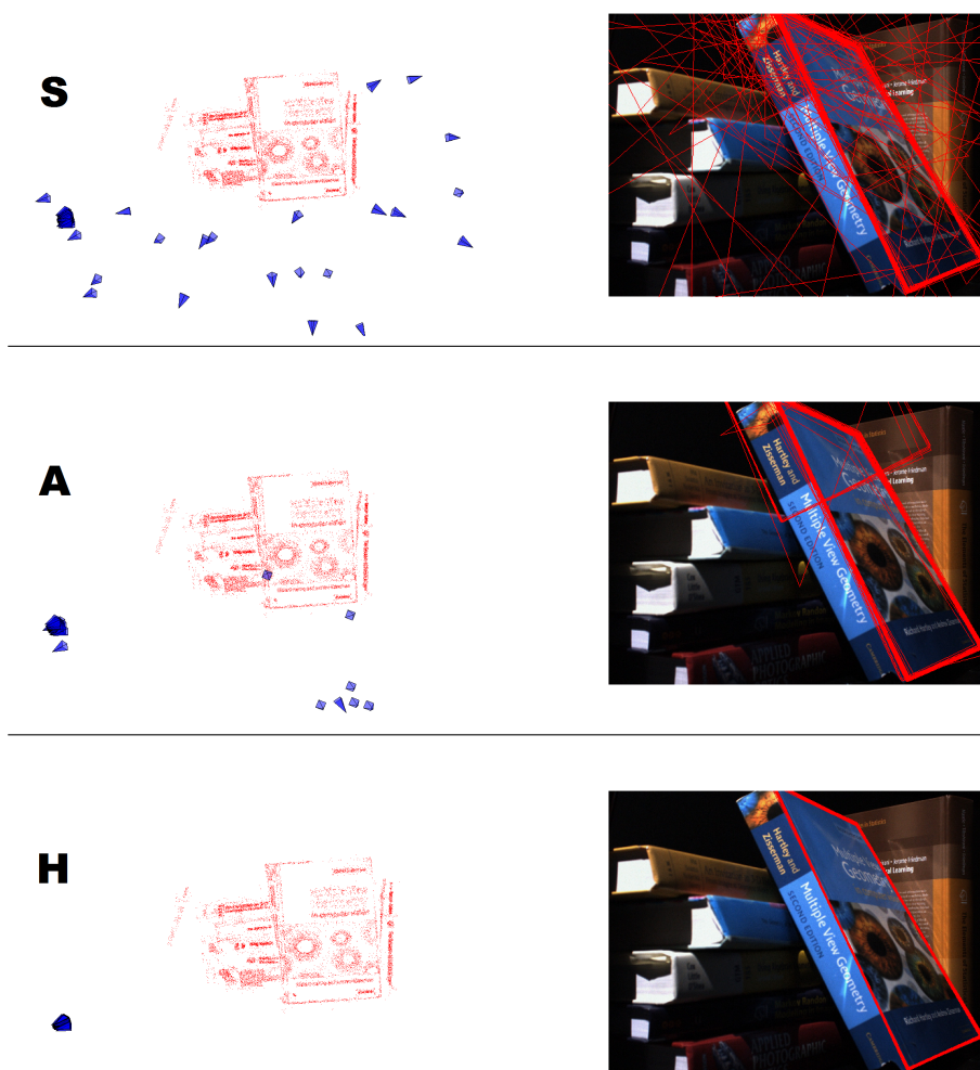
Figure 8. Séquence Livre : 100 poses calculées avec N = 500 itérations de RANSAC, et la reprojection des bords de la couverture en utilisant ces 100 poses. Dans le scénario H l'écart-type de la position de la caméra est 0,31% de la distance à la scène.
