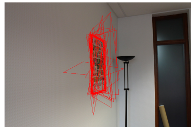
Figure 14. Séquence Mur : 100 calculs de pose avec N = 300 itération de RANSAC pour les trois vues de test (voir 13) dans le scénario S . De gauche à droite : les vues test 1 à 3. L'écart-type de la position de la caméra est 2,14% de la distance à la scène pour la vue 1 et 0,12% pour la vue 2
