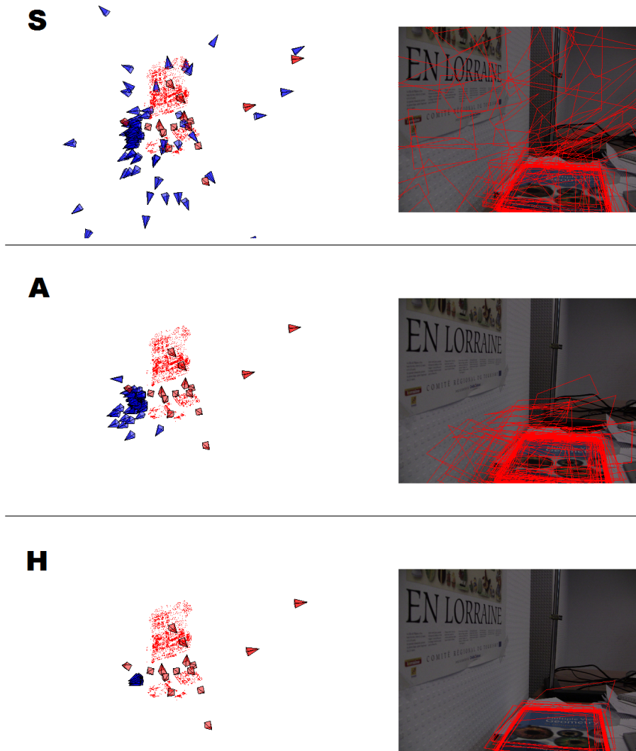
Figure 11. Séquence Bureau : 100 poses calculées avec N = 5000 itérations de RANSAC, et la reprojection des bords du livre de droite en utilisant ces 100 poses. Dans le scénario H l'écart-type de la position de la caméra est 3,04% de la distance à la scène.
