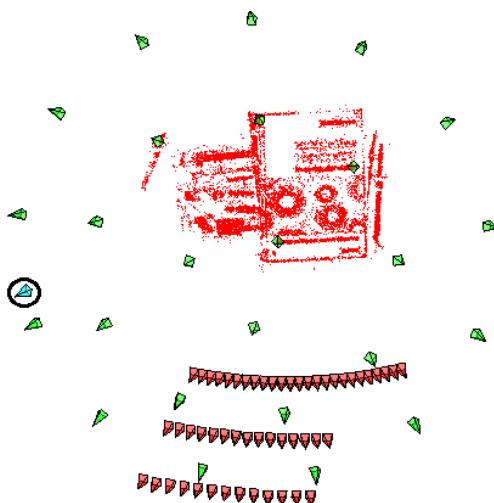
Figure 1. Le modèle 3D de la scène (points rouge), les caméras ayant servi à le construire (en rouge pâle), une caméra éloignée dont on chercherait la pose (en cyan, entouré), et les caméras virtuelles (en vert), réparties ici sur une demi-sphère. Les caméras virtuelles permettent de générer de nouveaux descripteurs pour chaque point du modèle.
