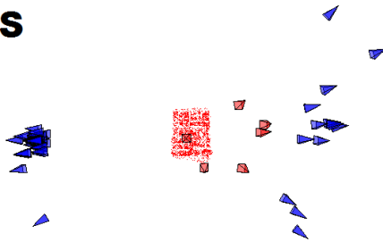
Figure 14. Séquence Mur : 100 calculs de pose avec N = 300 itération de RANSAC pour les trois vues de test (voir 13) dans le scénario S . De gauche à droite : les vues test 1 à 3. L'écart-type de la position de la caméra est 2,14% de la distance à la scène pour la vue 1 et 0,12% pour la vue 2
