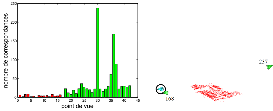
Figure 17. Séquence Poster : nombre de correspondances associées à chaque point de vue (réel en rouge, virtuel en vert), pour l'ensemble des correspondances image/modèle (à droite). Les deux points de vue correspondant aux pics dans l'histogramme sont un point de vue proche de la pose test et le point de vue symétrique (à droite ; les contributions respectives des deux points de vue sont indiquées).
