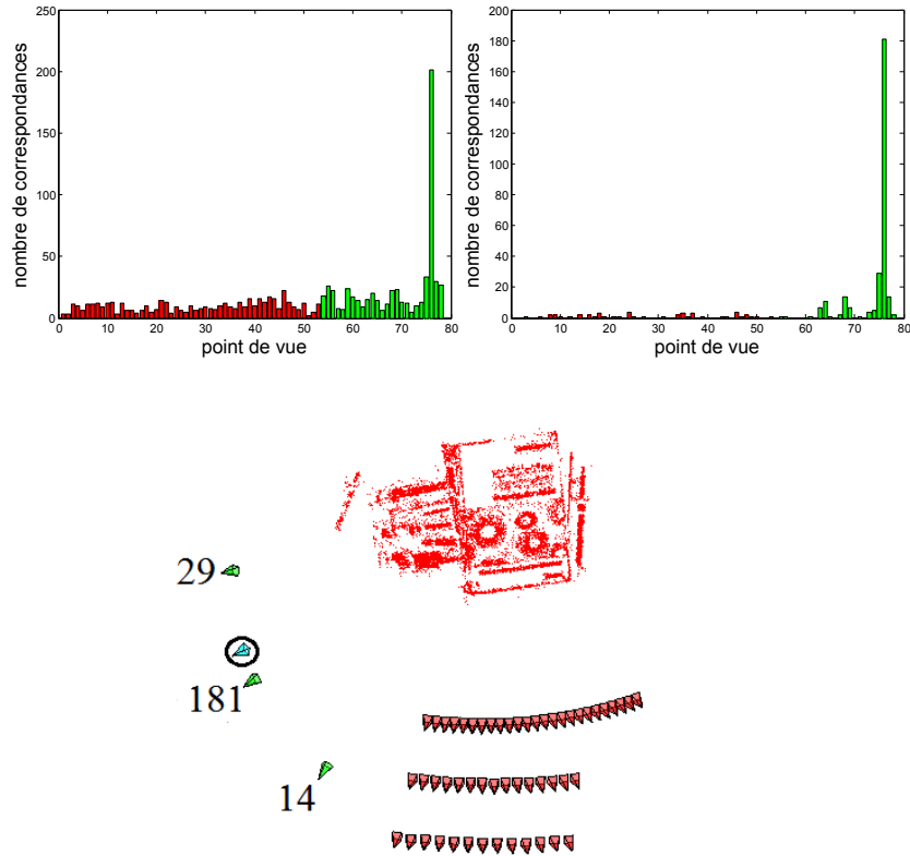
Figure 7. Séquence Livre : nombre de correspondances associées à chaque point de vue (réel en rouge, virtuel en vert), pour l'ensemble des correspondances image/modèle (en haut à gauche) et dans l'ensemble de consensus de RANSAC (en haut à droite). Les points de vue contribuant le plus restent les mêmes, et sont proches de la pose cherchée. Les trois points de vue contribuant le plus et le nombre de correspondances associées sont montrés en bas.
