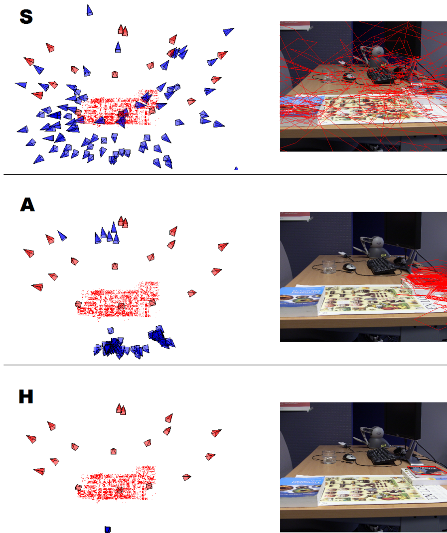
Figure 10. Séquence Poster : 100 poses calculées avec N = 1000 itérations de RANSAC, et la reprojection des bords du livre en utilisant ces 100 poses. Dans le scénario H l'écart-type de la position de la caméra est 0,07% de la distance à la scène.
