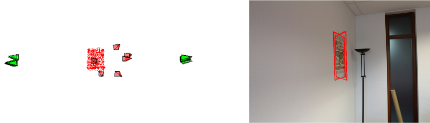
Figure 18. Séquence Mur : 100 calculs de pose avec N = 200 itérations de RANSAC pour la vue 3. Deux groupes de poses sont calculés, qui correspondent respectivement à la pose test (gauche) et à la position symétrique (droite).
